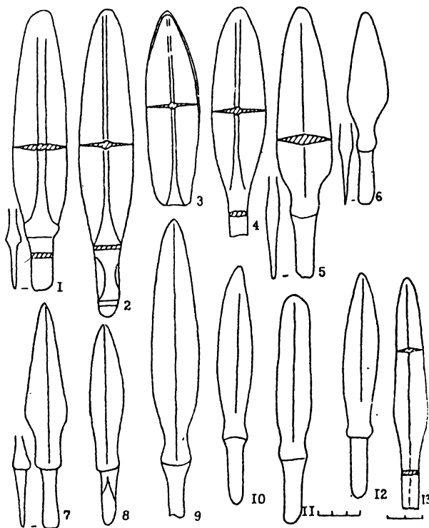
Рис. 54. Бронзовые кинжалы и нож: 1 — стоянка Ново-Кизгановская II; 2 — поселение Кузметово; 3 — поселение Бирское; 4 — Стерлибашевский краеведческий музей; 5, 6 — Кармановский клад; 7 — Красногорский I могильник; 8 — с. Катайское; 9 — оз. Малый Касаргуль; 10 — с. Кочневское; 11 — с. Куксянское; 12 — с. Троицкое; 13 — с. Березовское
