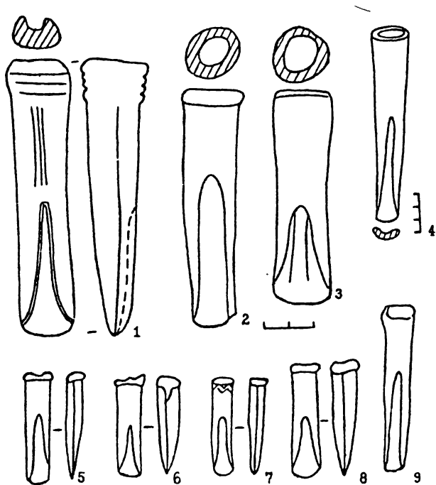
Рис. 49. Бронзовые долота: 1 — Дербедневский клад; 2 — поселение Черемуховый Куст; 3 — поселение Степное II; 4 — поселение Камышное II; 5 — поселение Луговское II; 6—7 — поселение Ананьинское; 8 — с. Ново-Мордово; 9 — Сосново-Мазинский клад
