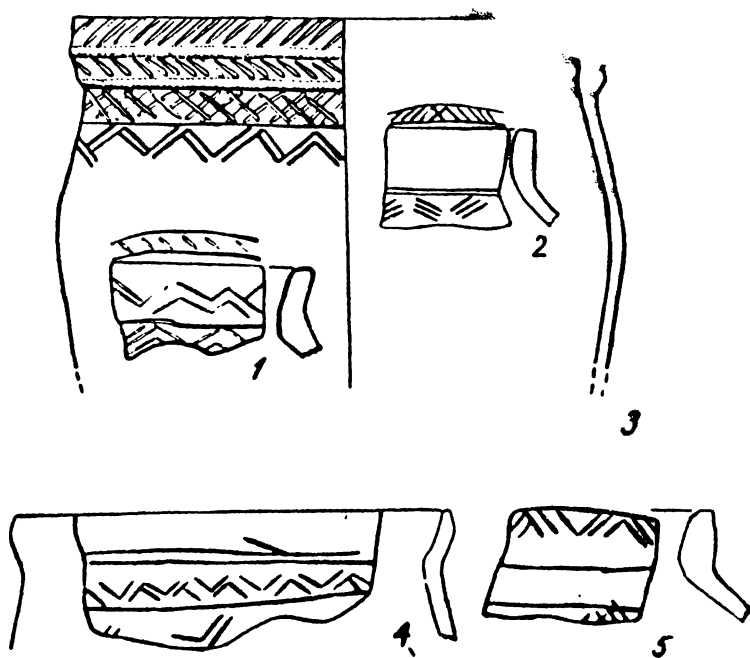
Рис. 38. Керамика межовского типа: 1 — поселение Перевозный III; 2 — поселение Березки V; 3—5 — поселение Аргазь XIII
