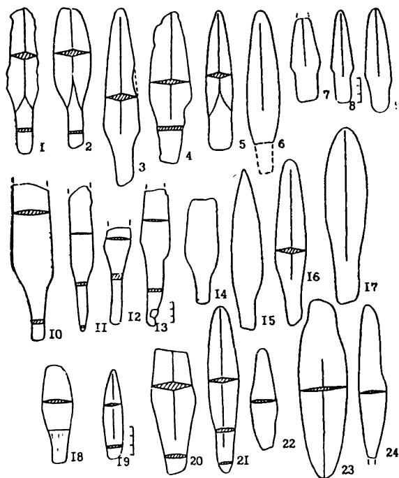
Рис. 53. Бронзовые ножи: 1, 2 — поселение Юкаликулево; 3, 18 — Такталачукский могильник, погребение 300; 4 — стоянка Старо-Кабановская II; 5 — поселение Шаблинское; 6, 7, 17 — Екатеринбургский историко-краеведческий музей; 8 — поселение Камышное I; 9 — поселение Криюши; 10 — стоянка Инзелга; 11 — поселение Таалыкаевское; 12 — поселение Лебяжье Островное; 13 — поселение Волостниковское; 14 — поселение Балымское, погребение I; 15 — поселение Чишминское; 16 — стоянка Березогривская I; 22 — поселение Кумысское; 23 — поселение Старо-Янгизитовское; 24 — поселение Зириковское
