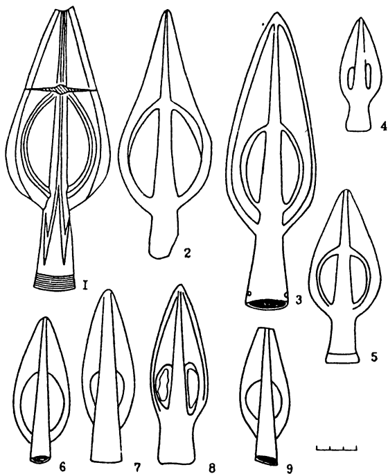
Рис. 56. Бронзовые кинжалы и наконечники стрел и копий: 1 — Кармановский клад; 2 — с. Тимашево; 3 — р. Миасс; 4 — оз. Карасий Исток; 5 — с. Пустобаево; 6 — с. Окольниково; 7 — Красногорский I могильник; 8 — Юмаковский могильник; 9 — оз. Ирбитское
