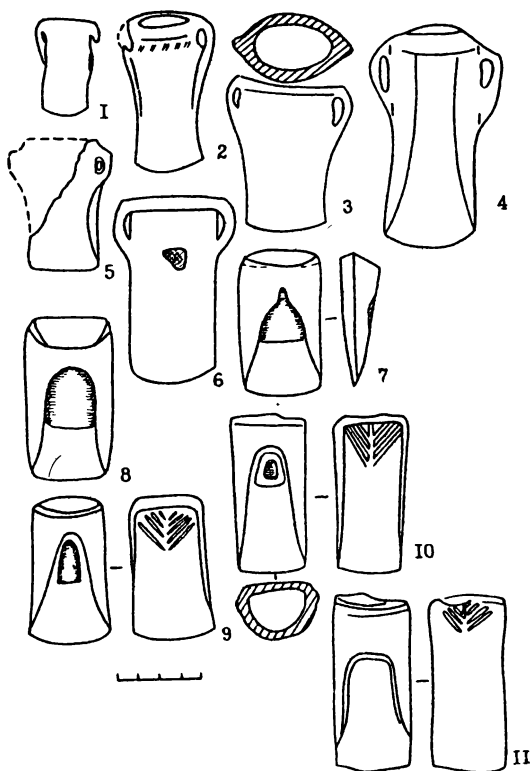
Рис. 47. Бронзовые кельты: 1 — городище Грохань; 2 — гора Петер-Тау; 3 — д. Сауз; 4 — д. Рысаево; 5 — поселение Усть-Бельское; 6 — Екатеринбургский историко-краеведческий музей; 7 — поселение Чесноковская Пашня; 8 — случ. нах. у р. Канащ; 9 — с. Китайское; 10 — с. Сулак; 11 — гора Нарис-Тау
