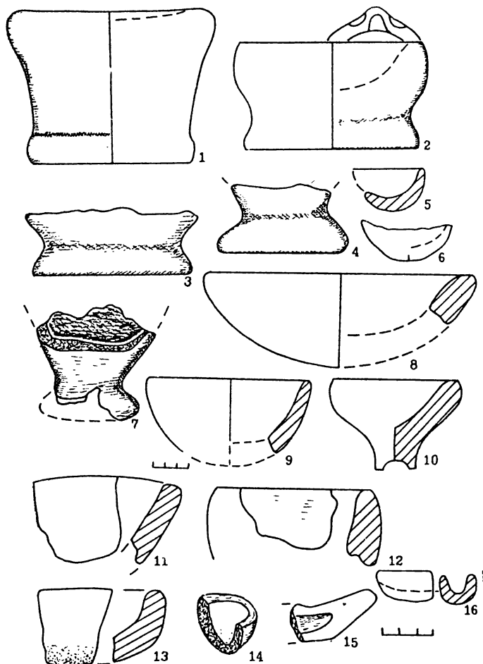
Рис. 63. Тигли и льячки: 1—3, 12—14 — поселение Тюбьяк; 4 — поселение Юкаликулево; 5 — стоянка Старо-Кабановская II; 6 — стоянка Кузькинская VII; 7 — д. Палкино (по В. Я. Толмачеву); 8 — стоянка Батрак-Айратовская; 9 — поселение Верхнее Биккузинское; 10 — Бирское поселение; 11 — поселение Нижегородское III; 15 — стоянка Старо-Яппаровская I; 16 — стоянка Старо-Яппаровская III
