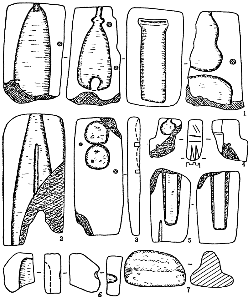
Рис. 61. Литейные формы и ложило: 1 — Башкирский краеведческий музей; 2 — стоянка Ахметовская I; 4, 5 — стоянка Дуванейская; 6 — поселение Нижегородское III; 7 — стоянка Кузькинская I; 1, 3, 4, 6 — камень; 2, 5, 7 — глина
