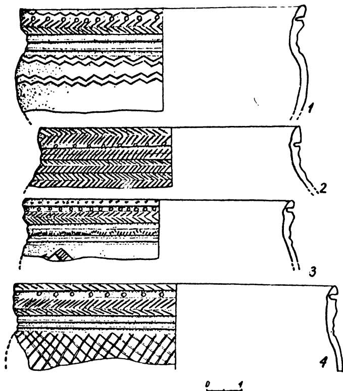
Рис. 35. Сосуды межовского типа. Поселение Кокшарово I
