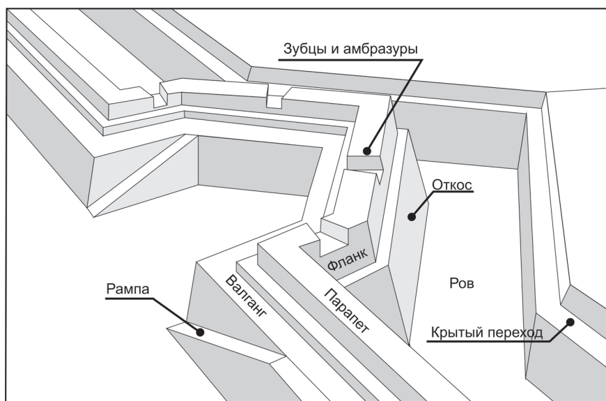
Рис.2. Схема оборонительного сооружения (на основе материалов [6])
